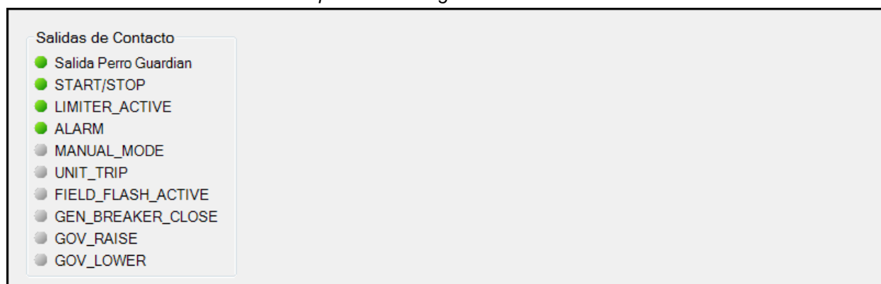
Figura 76. Pantalla de indicación del estado de las salidas de contacto del DECS-250E
