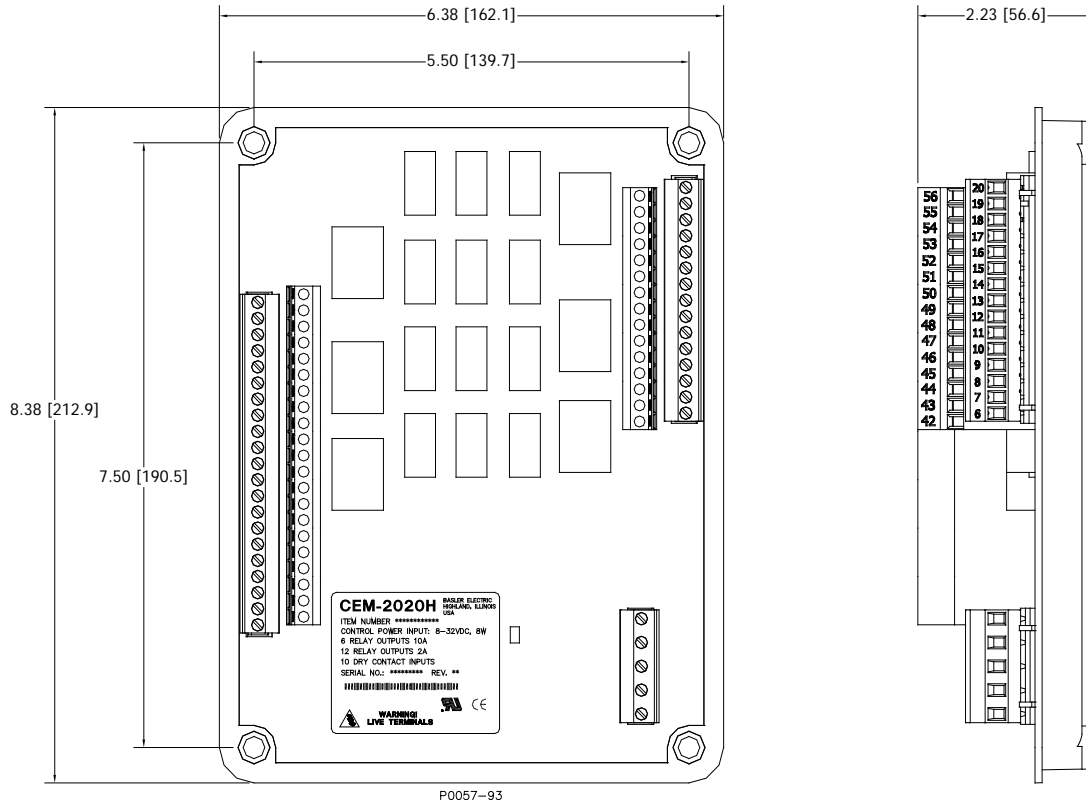
Figura 169. Dimensiones Generales del CEM-2020H
