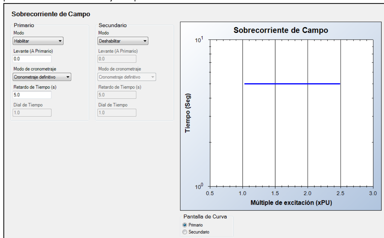
Figura 37. Ajustes de la protección de sobrecorriente de campo
