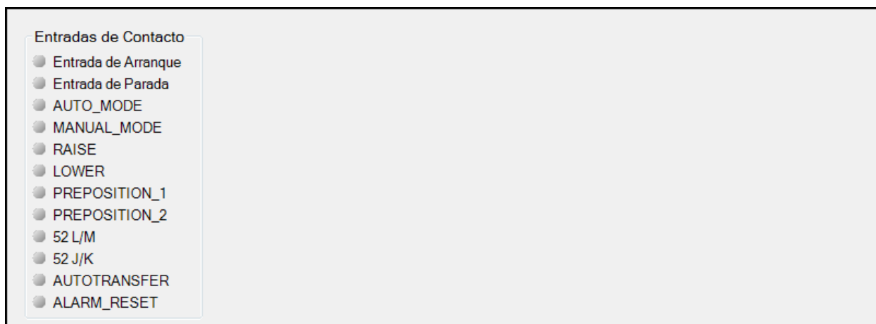
Figura 75. Pantalla de indicación del estado de las entradas de contacto del DECS-250E
