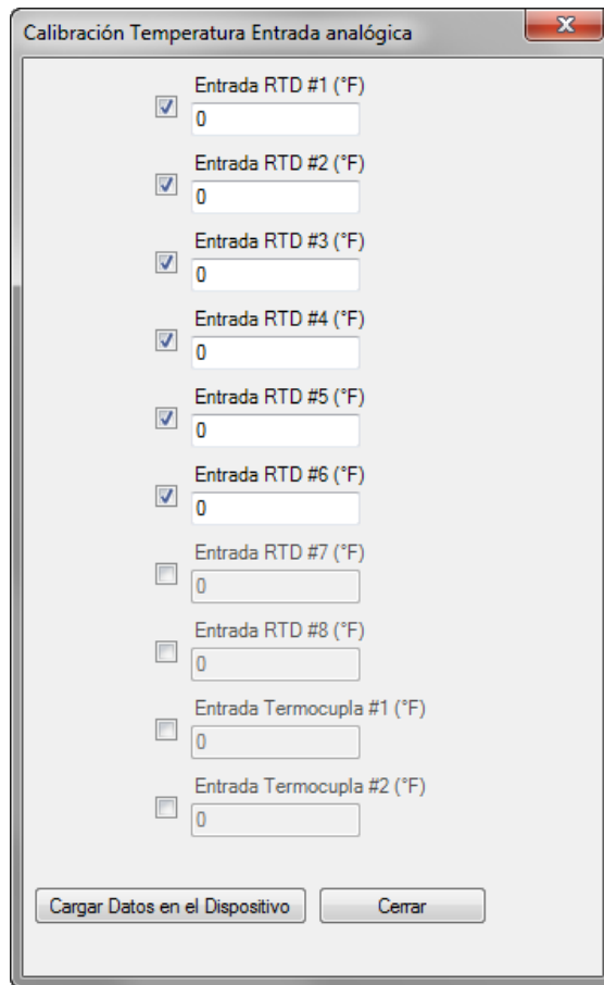
Figura 166. Calibración de la temperatura de la entrada analógica remota
