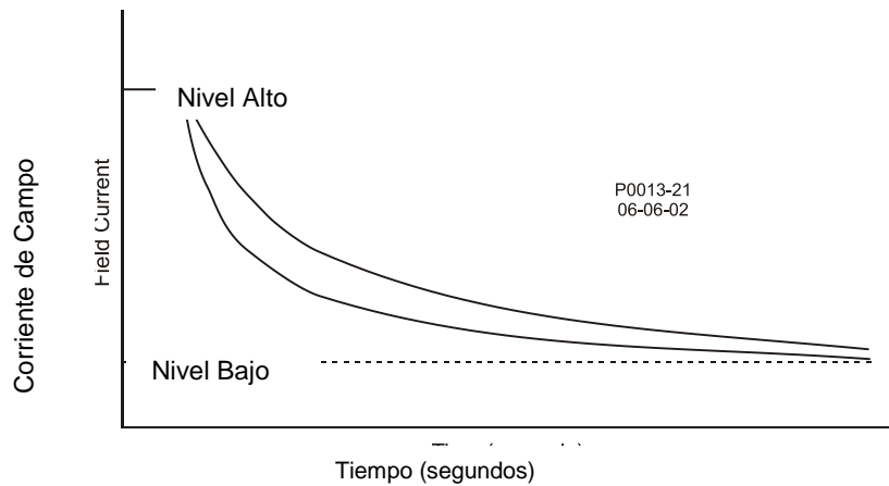
Figura 44. Características de tiempo inverso para Toma de Control OEL
