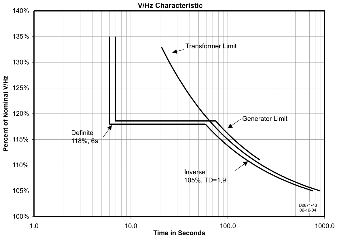
Figura 26. Característica de V/Hz (el tiempo se muestra en el eje horizontal)
