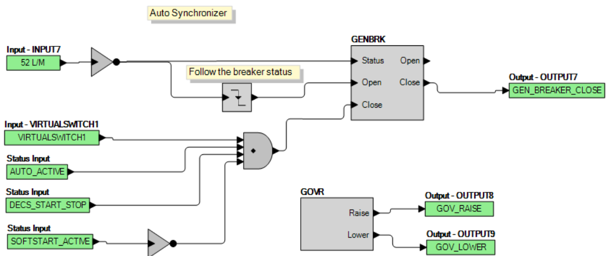
Figura 112. Lógica predeterminada habilitada de sincronizador automático - Pestaña Página de lógica 3
