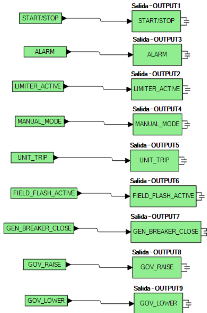
Figura 113. Lógica predeterminada de sincronizador automático - Pestaña Salidas físicas
