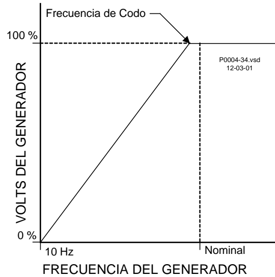
Figura 18. Curva de Compensación de Subfrecuencia Típica
