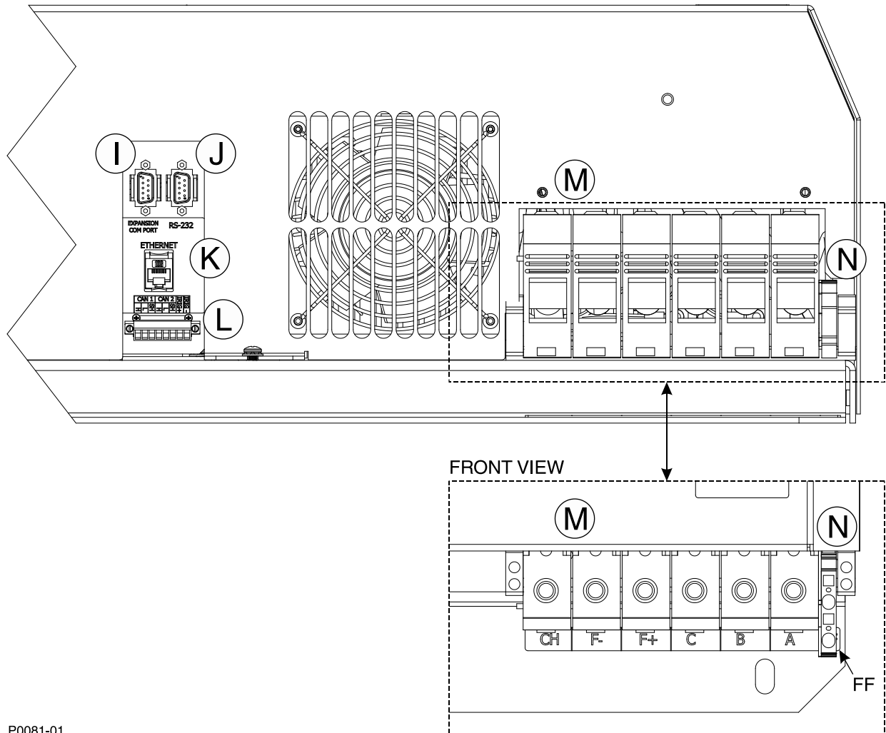
Figura 5. Conectores y terminales inferiores
