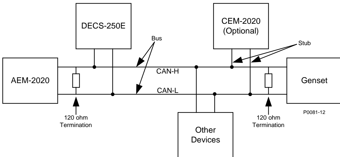
Figura 156. Interfaz de CAN Bus con AEM-200 proporcionando Un Extremo del Bus
