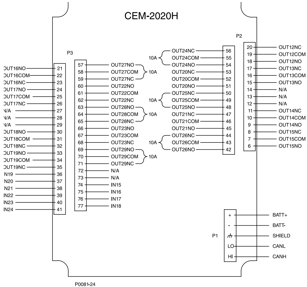
Figura 171. Terminales de Contacto de Salida y Contacto de Entrada del CEM-2020H
