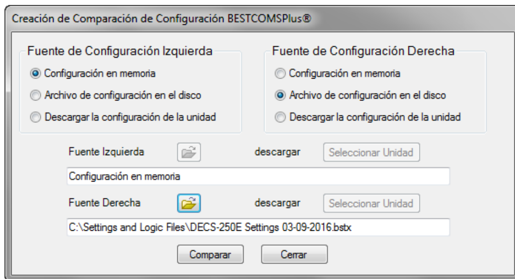
Figura 103. Configuración de comparación de ajustes de BESTCOMSP Plus
