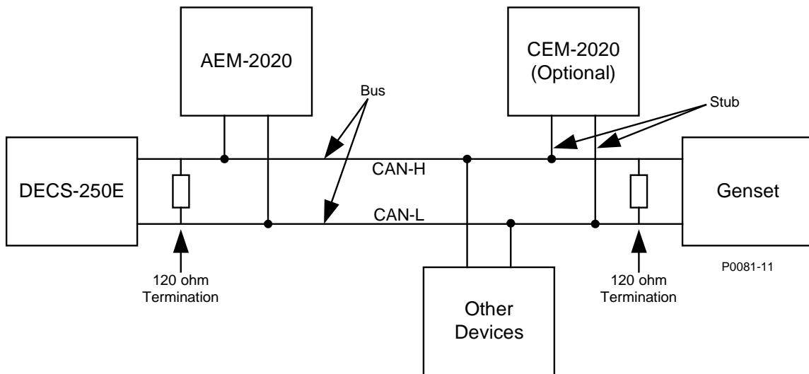
Figura 155. Interfaz del bus de la CAN con el DECS-250E que brinda un extremo del bus
