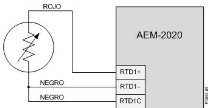
Figura 154. Conexiones de Entrada RTD Externas de tres hilos
