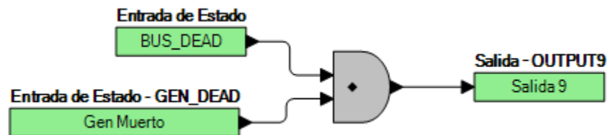
Figura 118. Ejemplo 2: Conexiones de compuerta AND
