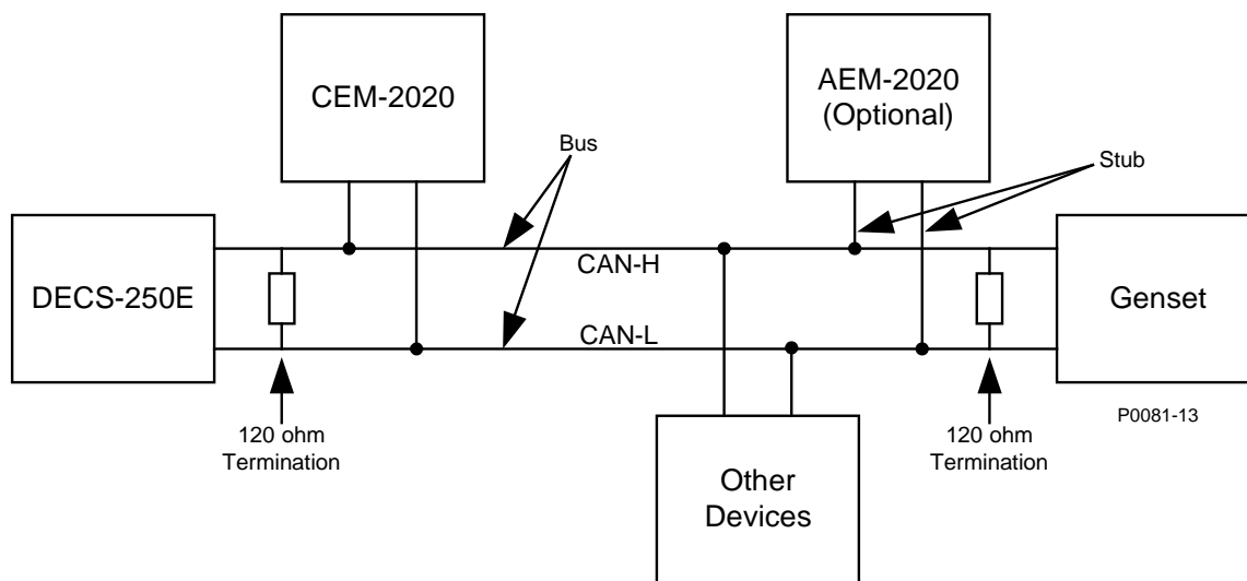
Figura 172. Interfaz del bus de la CAN con el DECS-250E, que brinda un extremo del bus
