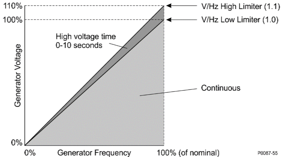
Figura 19. Curva típica del Limitador de 1.1 PU Voltios por Hertzio
