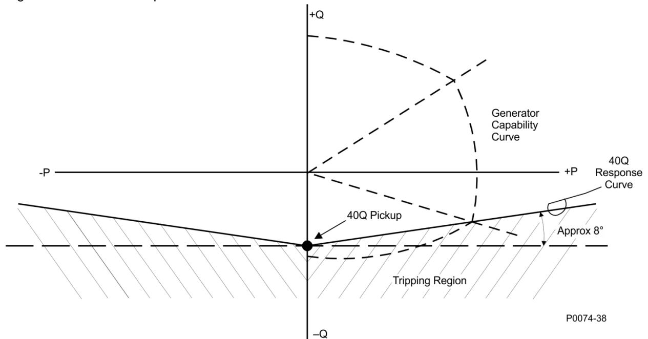
Figura 34. Curva de capacidad del generador frente a la respuesta de 40Q
