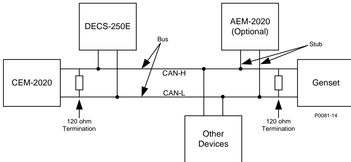
Figura 173. Interfaz del bus de la CAN con el CEM-200, que brinda un extremo del bus
