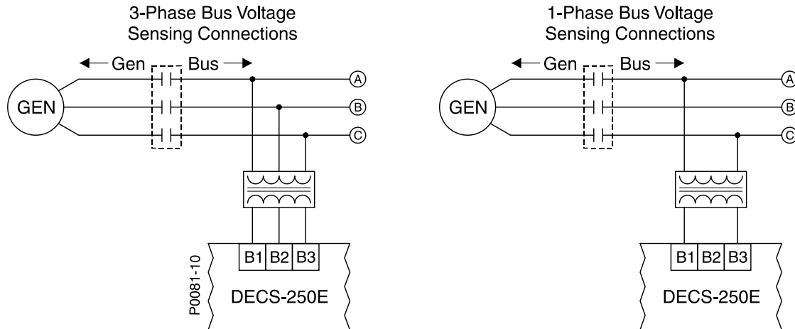
Figura 15. Conexiones Típicas de la Medición de Tensión del Bus
