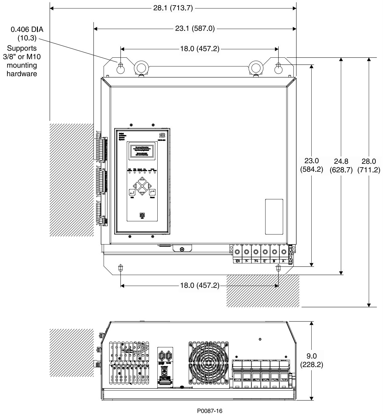
Figura 3. Dimensiones generales y del montaje
