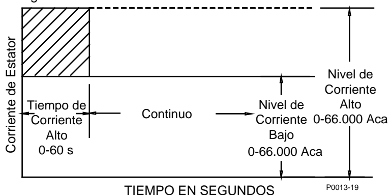
Figura 14. Limitador de Corriente Estatórica
