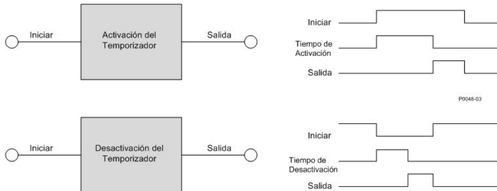
Figura 114. Bloques de la Lógica de Temporizador de Activación y Caída
