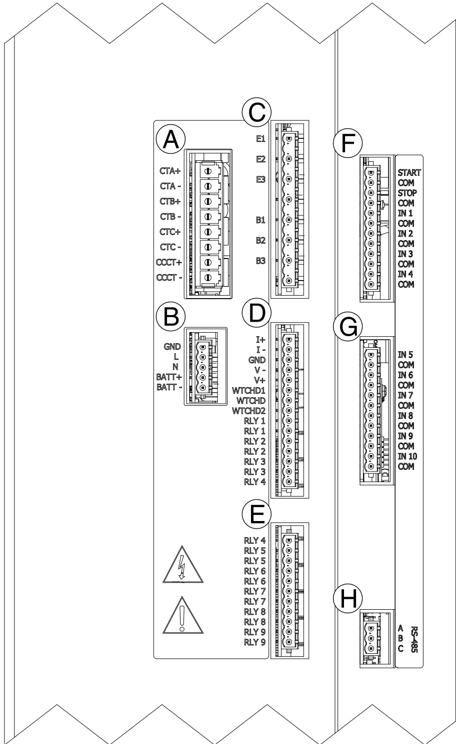
Figura 4. Terminales del panel izquierdo
