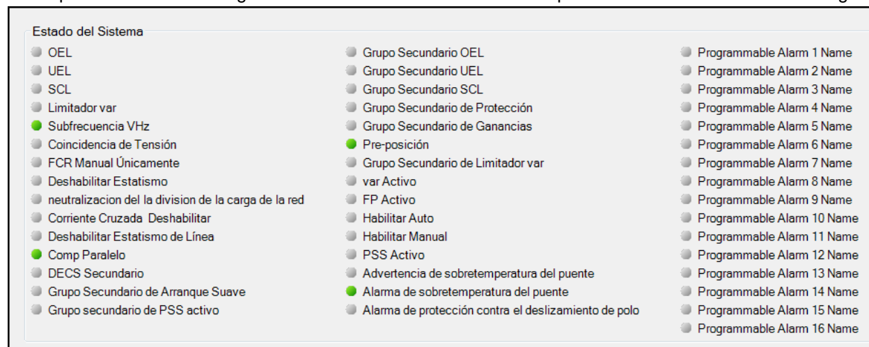
Figura 74. Pantalla de indicación Estado del sistema
