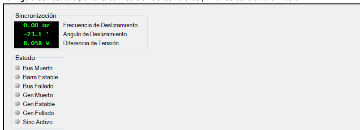
Figura 69. Medición de valores primarios de la sincronización
