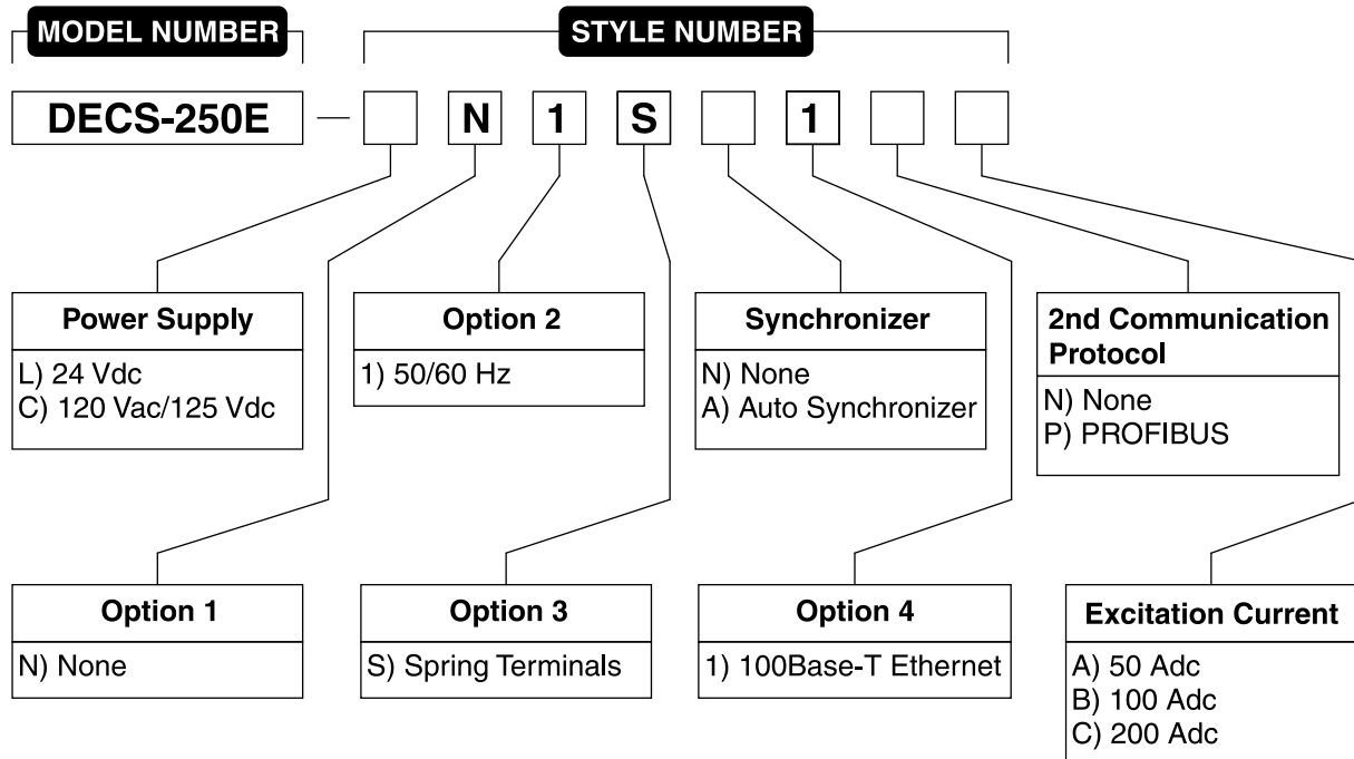
Figura 1. Tabla de estilos del DECS-250E
