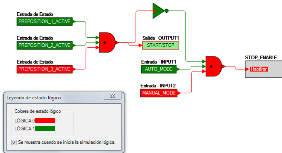
Figura 115. Ejemplo del simulador de lógica fuera de línea
