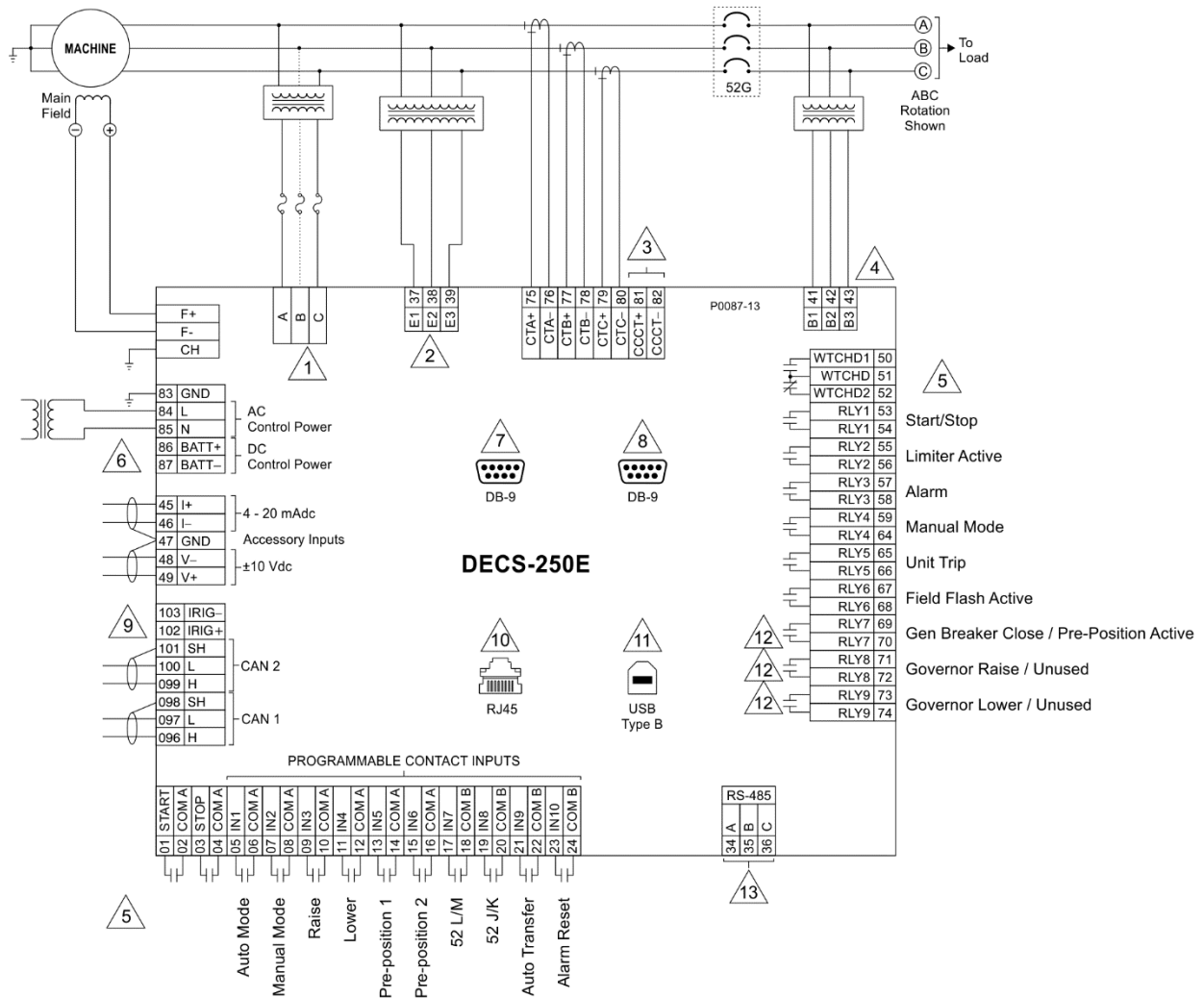
Figura 6. Conexiones de DECS-250E típicas para las aplicaciones accionadas por derivación
