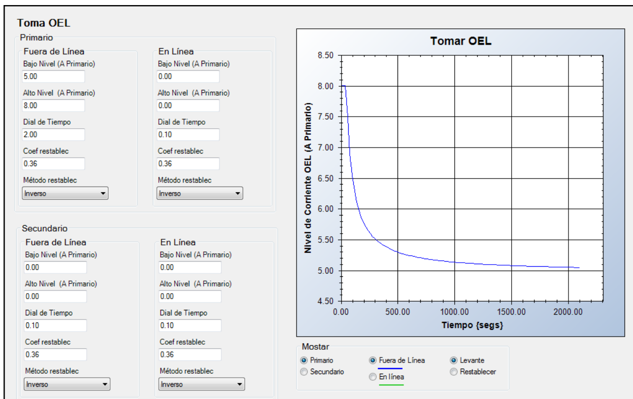
Figura 11. Ajustes de OEL de sustitución
