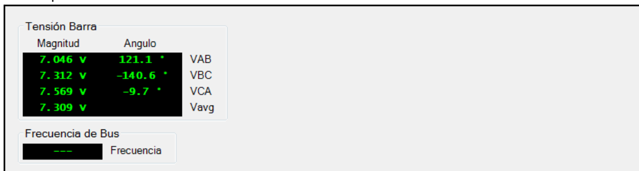
Figura 67. Medición de valores primarios del bus
