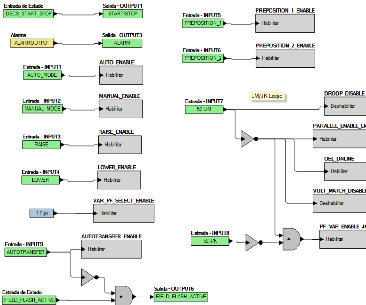
Figura 108. Lógica predeterminada – Pestaña Página de lógica 1
