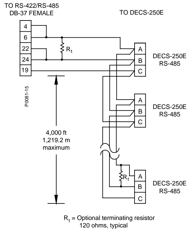
Figura 121. Conexiones típicas de RS-485
