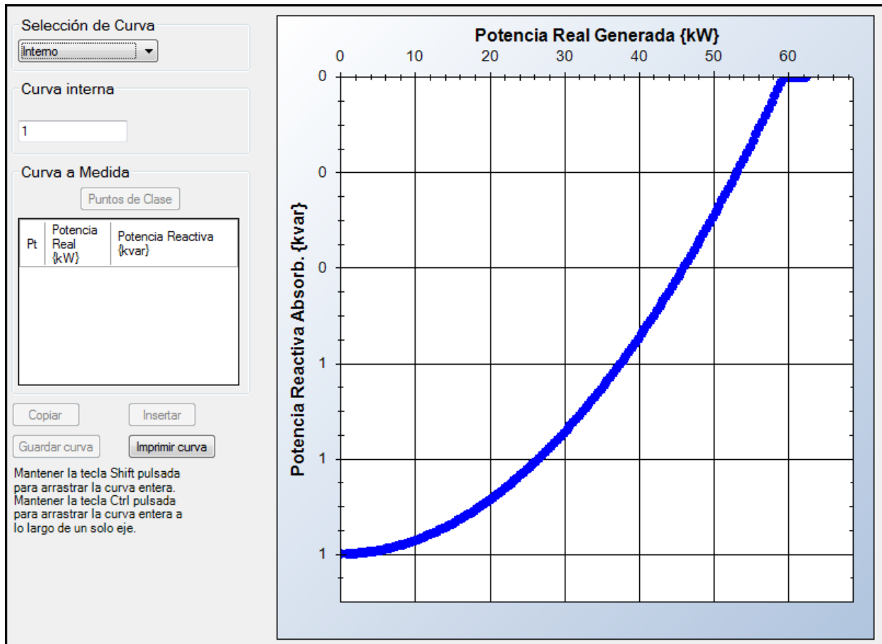
Figura 13. Pantalla de la curva personalizada primaria de UEL
