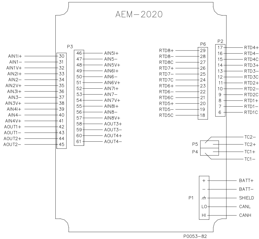
Figura 150. Terminales de Entrada y Salida
