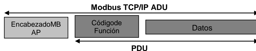
Figura 148. Petición/Respuesta de Modbus en TCP/IP
