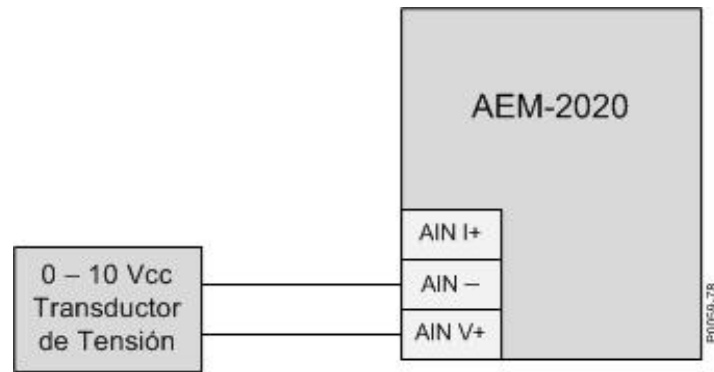
Figura 151. Entradas Analógicas – Conexiones de Entrada de Tensión
