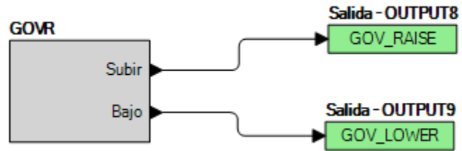
Figura 117. Ejemplo 1 - Conexiones del Bloque Lógico del GOBERNADOR
