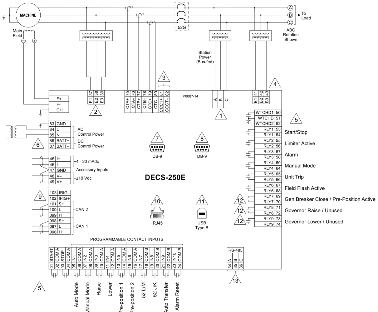
Figura 7. Conexiones de DECS-250E típicas para las aplicaciones accionadas por PMG
