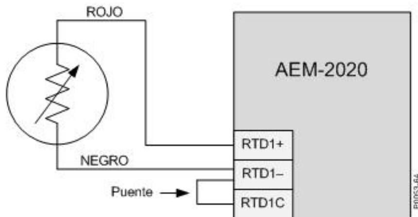
Figura 153. Conexiones de Entrada RTD Externas de dos hilos
