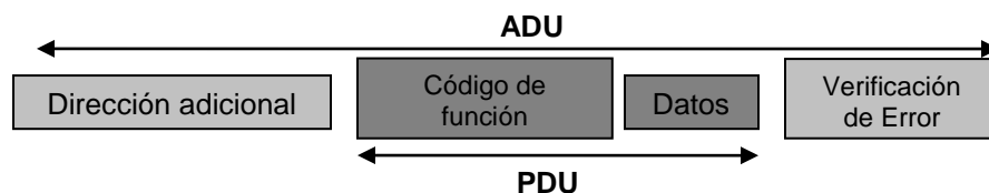
Figura147. Marco General del Modbus
