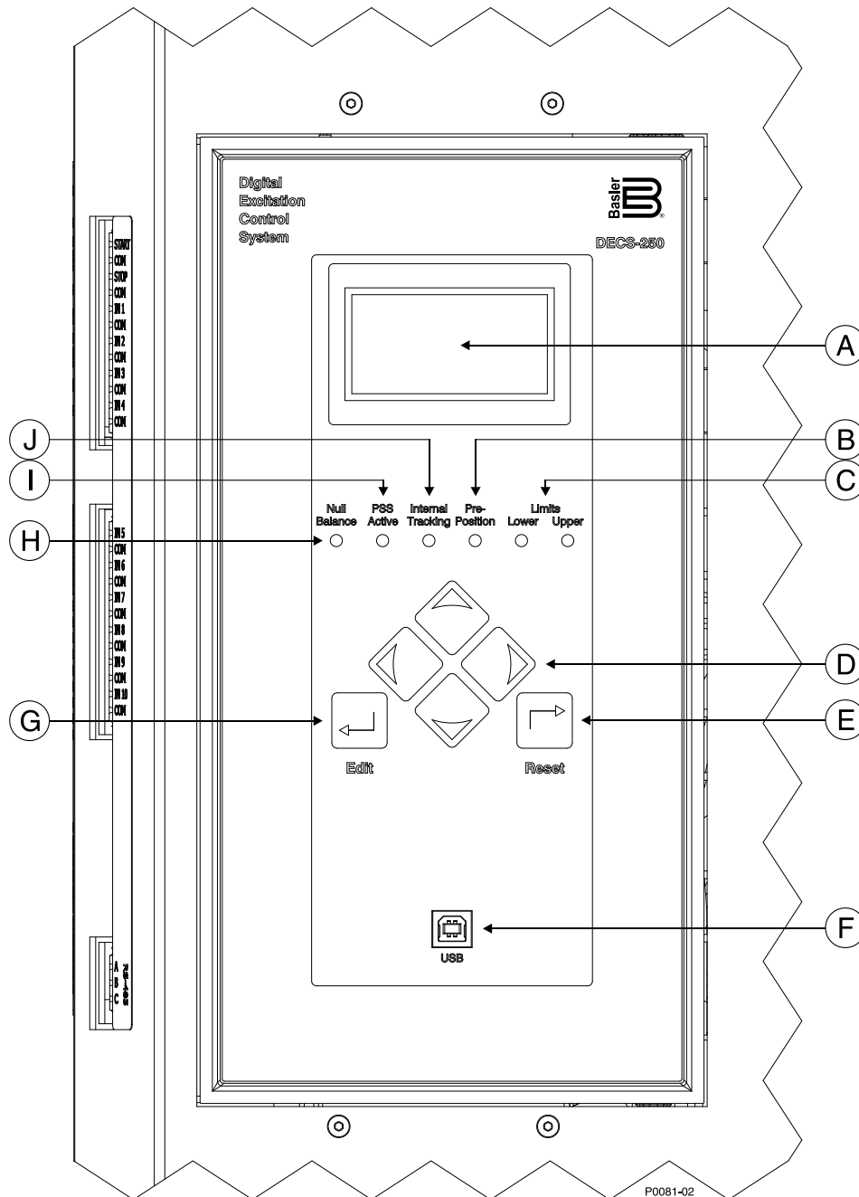
Figura9. Controles e Indicadores del Panel Frontal
