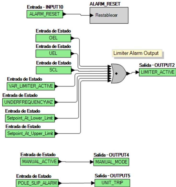
Figura 111. Lógica predeterminada habilitada de sincronizador automático - Pestaña Página de lógica 2
