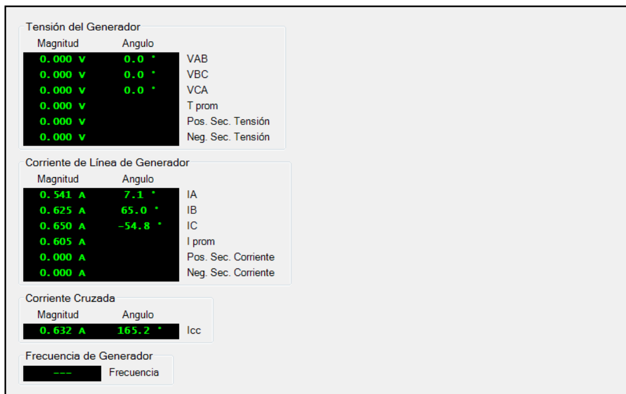
Figura 64. Medición de valores primarios del generador
