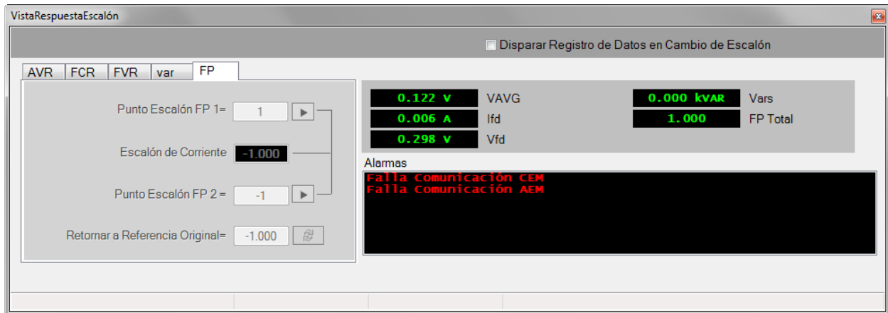
Figura 144. Análisis de Respuesta de Escalón - Tab PF
