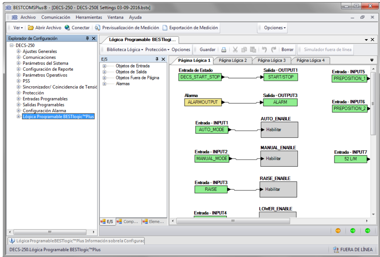
Figura 107. Rama del árbol Lógica programable de BESTlogicPlus
