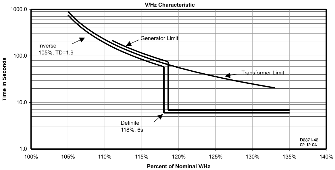
Figura 25. Característica de V/Hz (el tiempo se muestra en el eje vertical)
