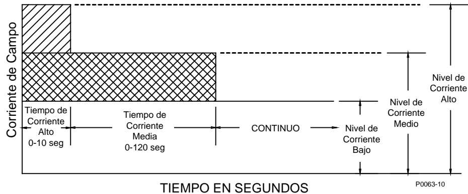
Figura 43. Punto de Suma, Online, Limitador de Sobreexcitación
