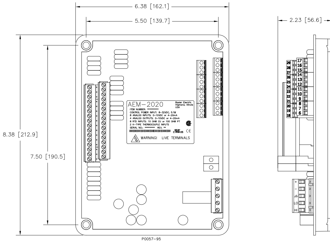
Figura 149. Dimensiones Generales del AEM-2020
