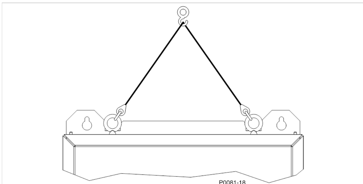
Figura 2. Diagrama de elevación
