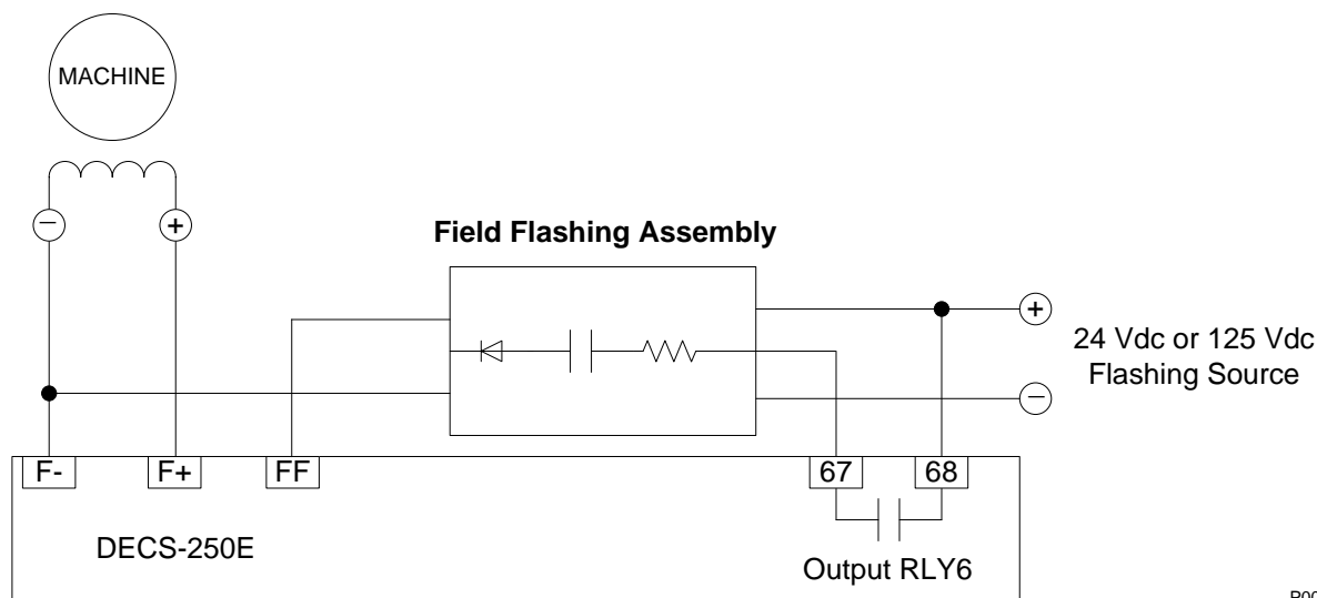
Figura 8. Conexiones típicas para el centelleo de campo
