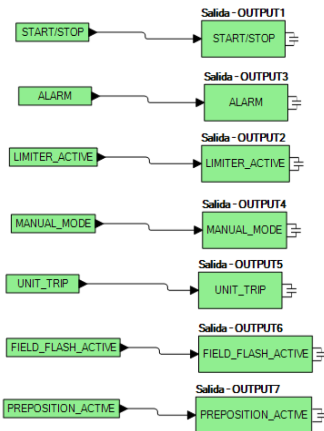
Figura 110. Lógica predeterminada - Pestaña Salidas físicas
