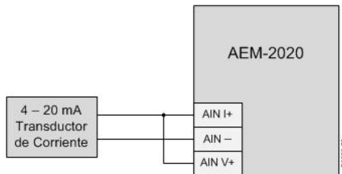
Figura 152. Entradas Analógicas – Conexiones de Entrada de Corriente
