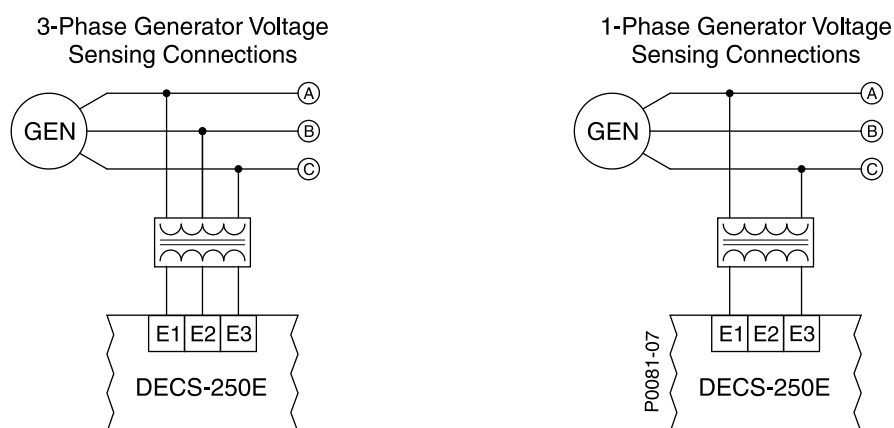
Figura 12. Conexiones Típicas de Medición de Tensión del Generador.
