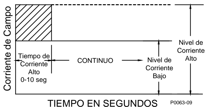
Figura 42. Punto de Suma, Sin conexión, Limitador de Sobreexcitación
